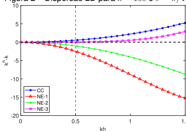
Figura 2 – Dispersão 2D para k = 100 e \theta = \pi/4
