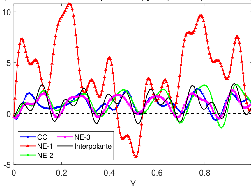
Figura 7 – Soluções numéricas 2D na seção x = 0.5 , f = 0 , k = 100 , kh = 0.5 e \theta_i = \{0, \pi/4, \pi/8\}
