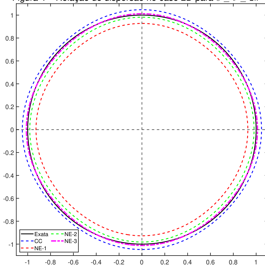
Figura 4 – Relação de dispersão no caso 2D para 0 \leq \theta \leq 2\pi
