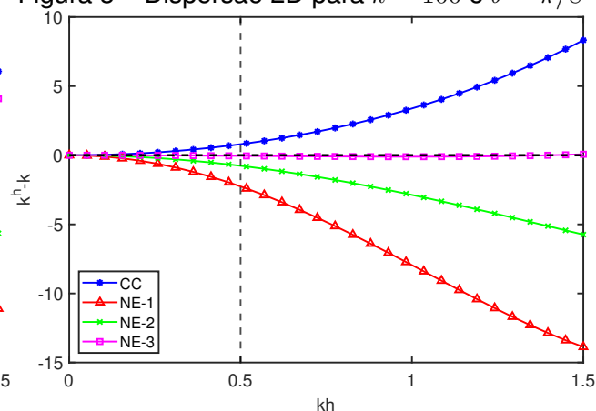
Figura 3 – Dispersão 2D para k = 100 e \theta = \pi/8
