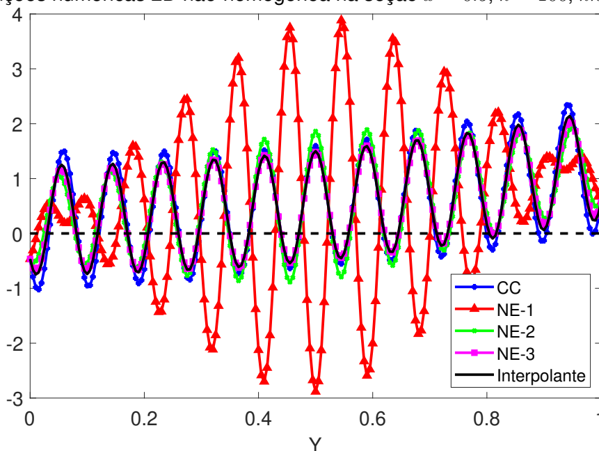
Figura 9 – Soluções numéricas 2D não-homogênea na seção x = 0.5 , k = 100 , kh = 0.5 e \theta = \pi/4
