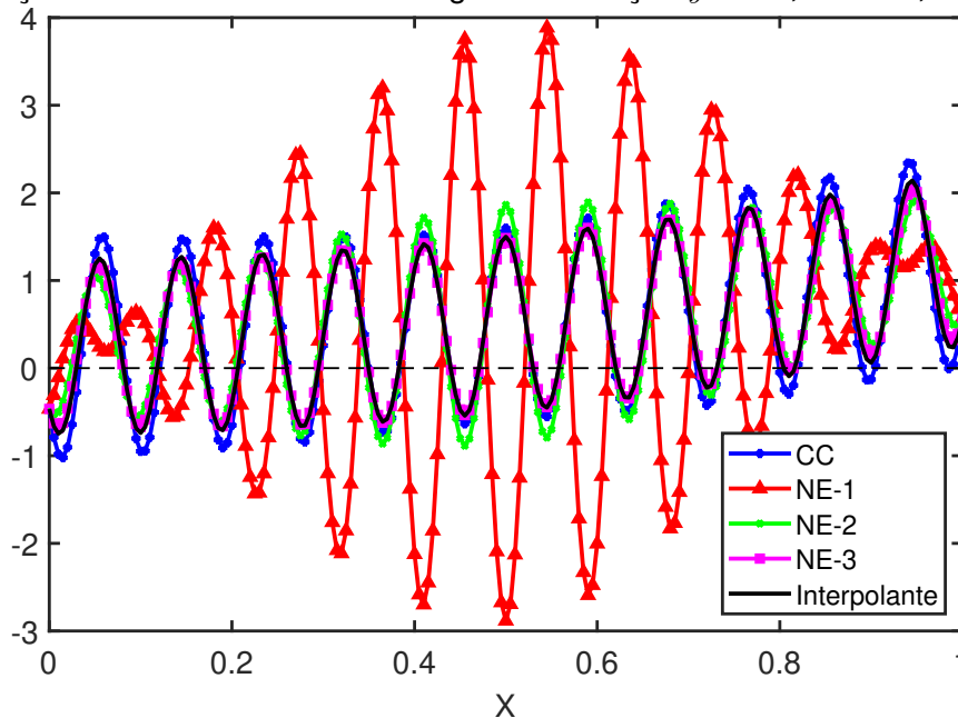
Figura 10 – Soluções numéricas 2D não-homogênea na seção y = 0.5 , k = 100 , kh = 0.5 e \theta = \pi/4
