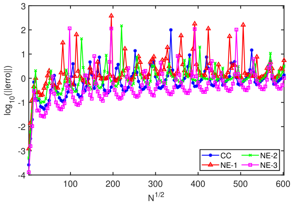
Figura 6 – Erro no caso 2D mantendo-se kh = 0.5 constante com k variando de 1 a 300 e \theta = \pi/4
