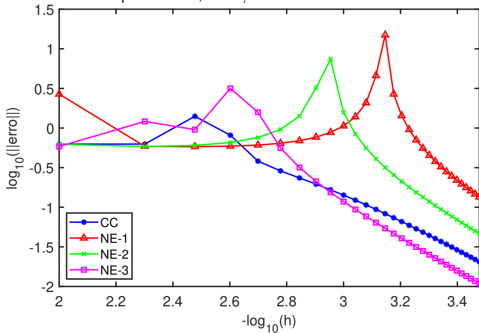
Figura 5 – Erro no caso 2D para k = 80 , \theta = \pi/4 e variando-se N de 100 \times 100 a 3000 \times 3000
