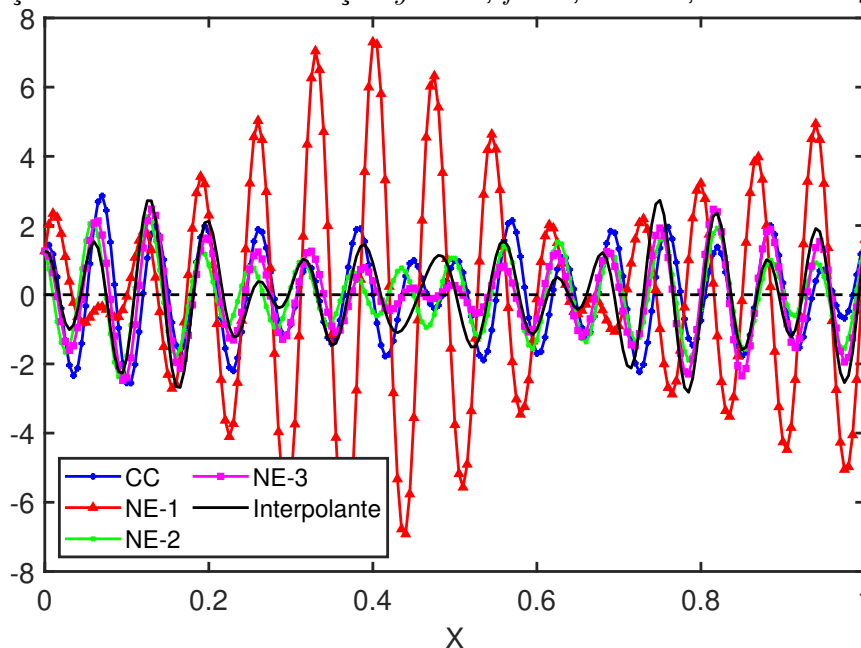
Figura 8 – Soluções numéricas 2D na seção y = 0.5 , f = 0 , k = 100 , kh = 0.5 e \theta_i = \{0, \pi/4, \pi/8\}
