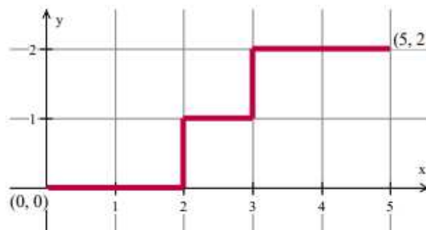
Figura 1: Exemplo de um caminho no retângulo 5 por 2
