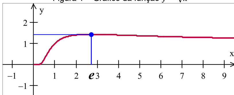
Figura 1 – Gráfico da função y = x^{\frac{1}{x}}
