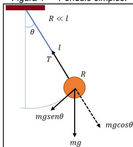
Figura 1 – Pêndulo simples.
